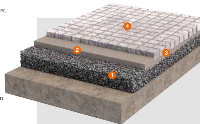
System Pflaster mit drainfähigem Fugenmörtel
