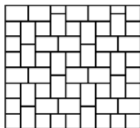
Suave 2 Kreuzverband Bedarf pro m 2 : 19,6 Stk. - 24/16/6 9,8 Stk. - 16/16/6
