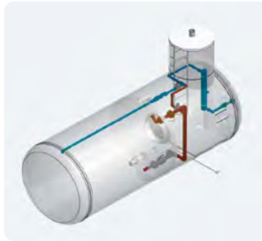
Speicher mit UV-Entkeimung
