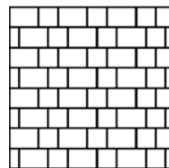
Suave 5 Gotischer Verband Bedarf pro m 2 : 15,6 Stk. - 24/16/6 15,6 Stk. - 16/16/6
